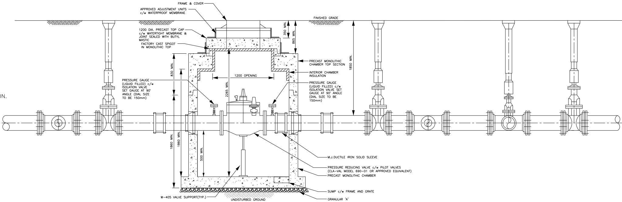
SECTION A-A
