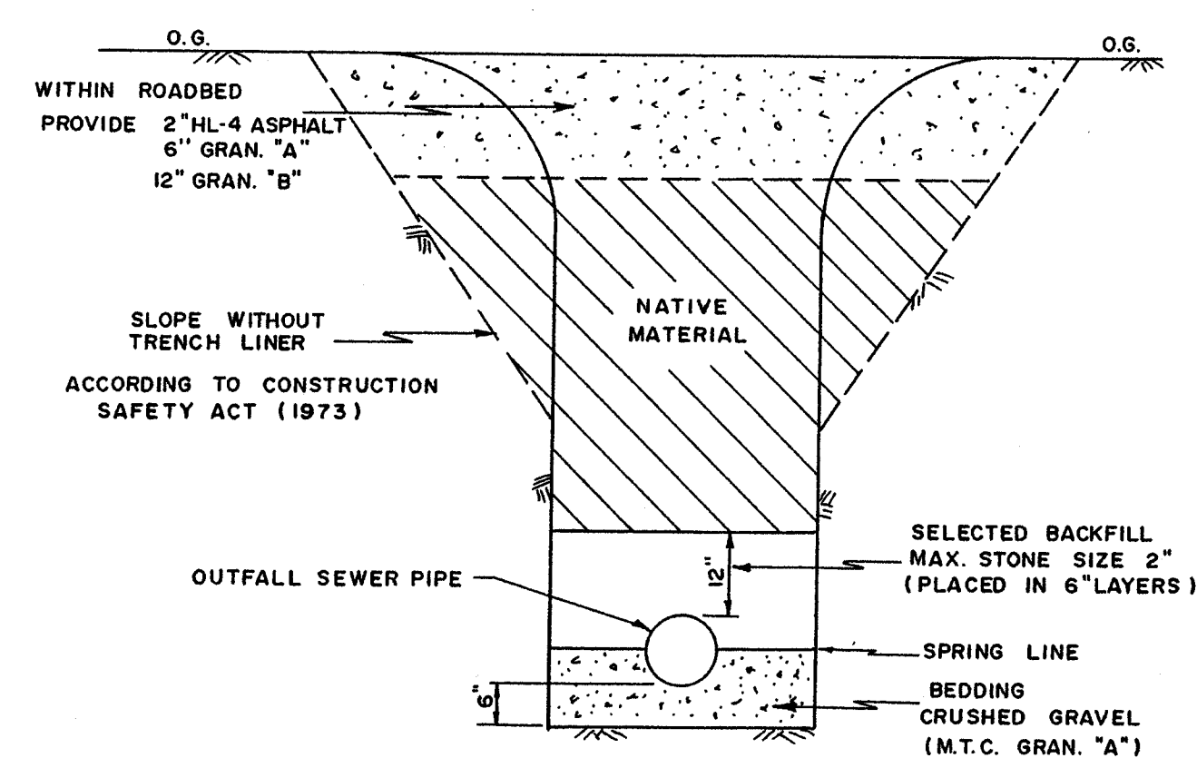
SECTION THROUGH OUTFALL SEWER STA. 4+50 TO STA. 9+50 ± N. T. S.
